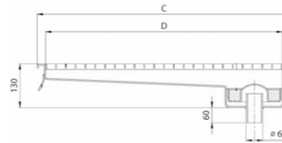
Flow system with grating Standard Ablaufsystem mit Gitterrost Standard Sistemi di drenaggio grigliati Standard A 300-500 B 250-450 D 1000-3000
