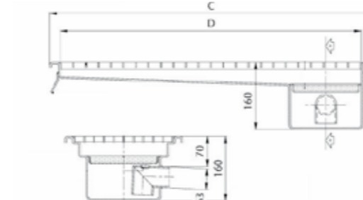
Flow system with grating Standard Ablaufsystem mit Gitterrost Standard Sistemi di drenaggio grigliati Standard A 300-500 B 250-450 D 1000-3000
